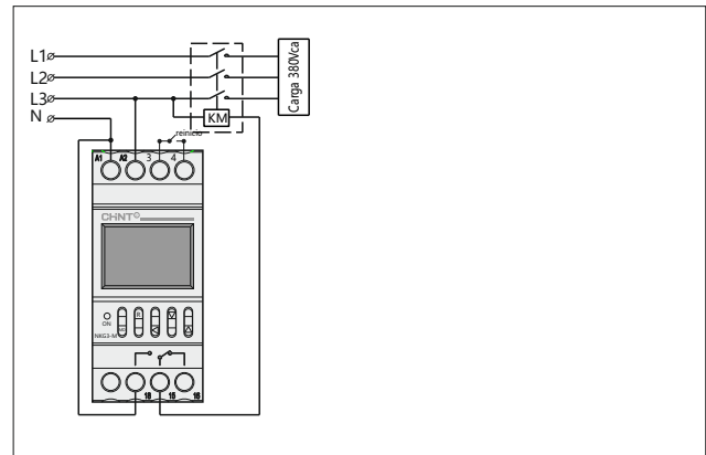
Imagen 4 Diagrama de conexión de control trifásico (bobina del contactor: 220V)
