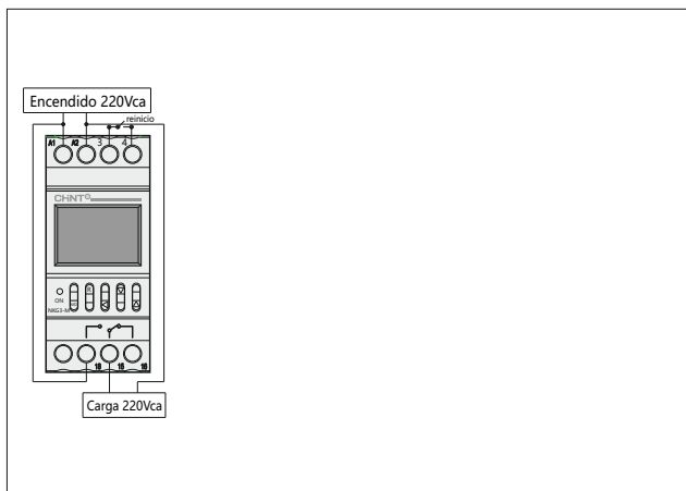
Imagen 1 Diagrama de conexión de control directo monofásico
