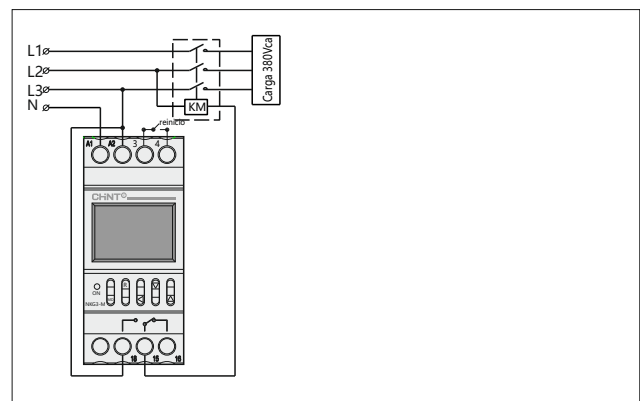
Imagen 5 Diagrama de conexión de control trifásico (bobina del contactor: 380V)
