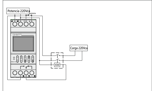
Imagen 2 Diagrama de conexión de control de expansión monofásica (bobina del contactor: 220V)
